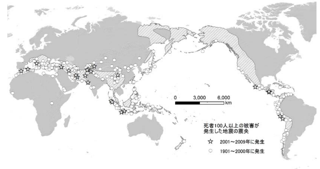
図2 世界の地震分布
