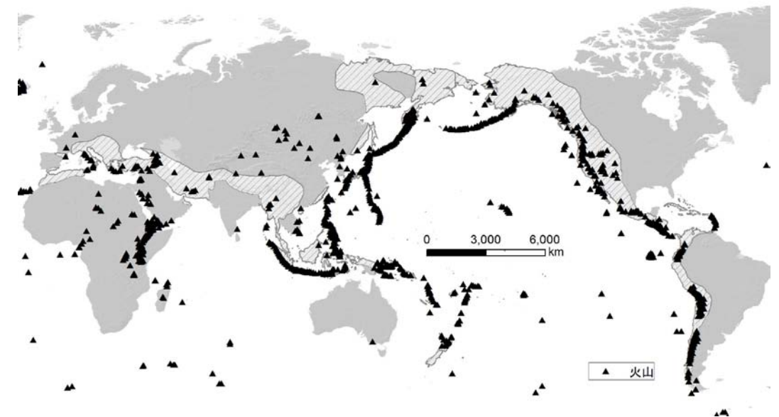
図3 世界の火山分布
