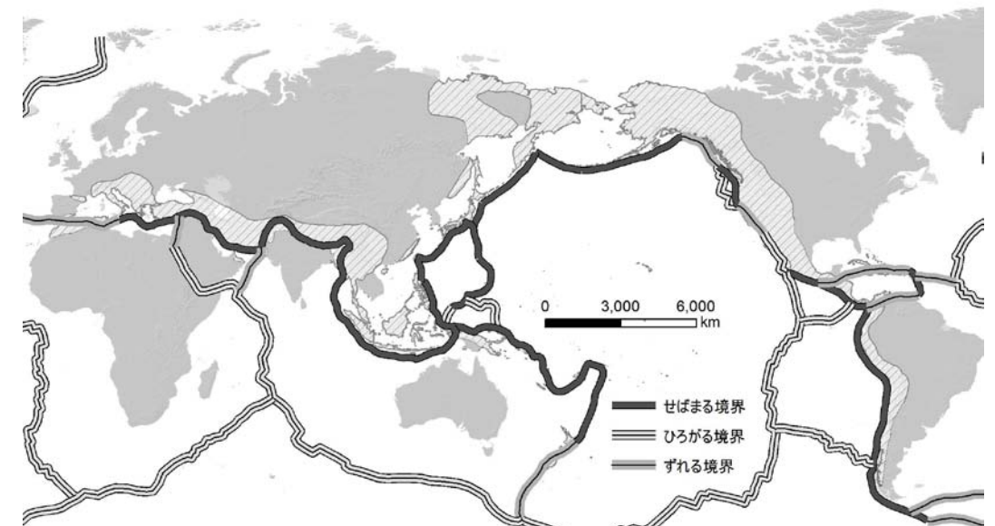
図4 世界のプレート境界
