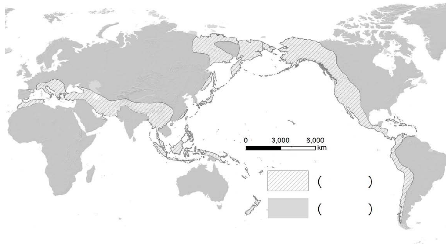
図1 世界の大地形
