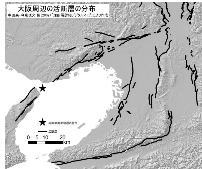
図3 大阪周辺の活断層の分布
