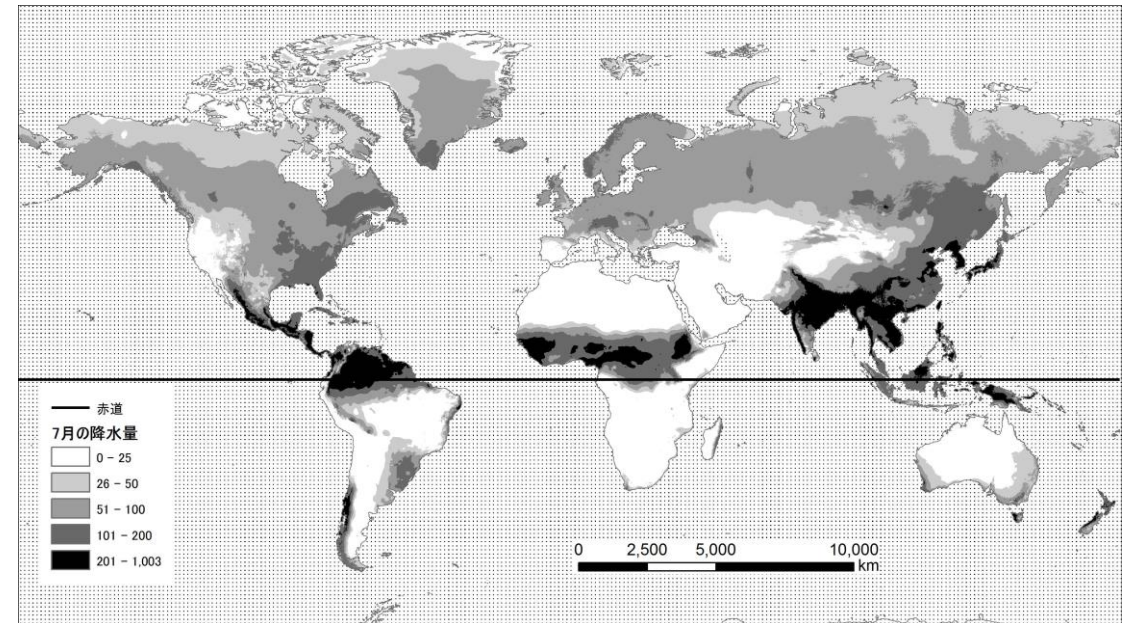
図5 世界の7月の降水量分布
