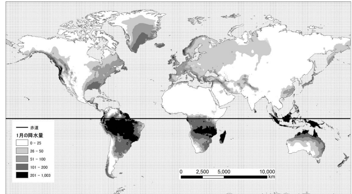
図6 世界の1月の降水量分布
