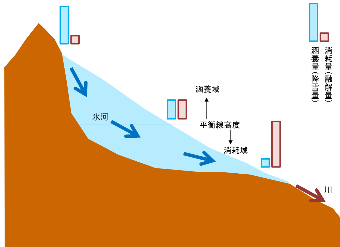
図3 氷河の質量収支
