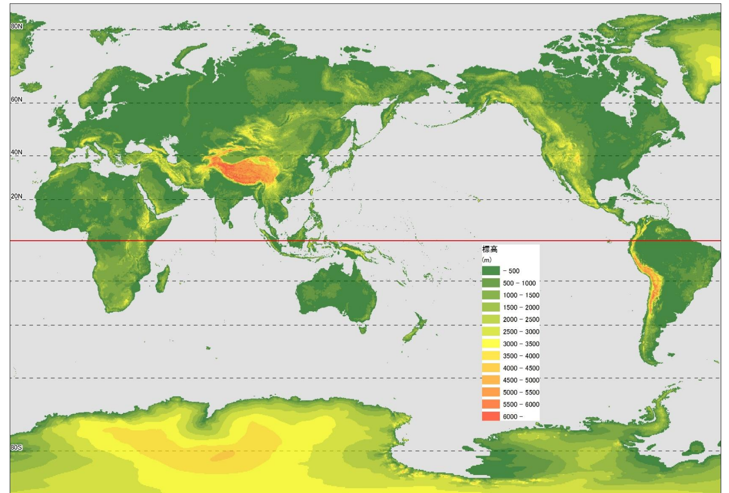
図2 標高の分布
