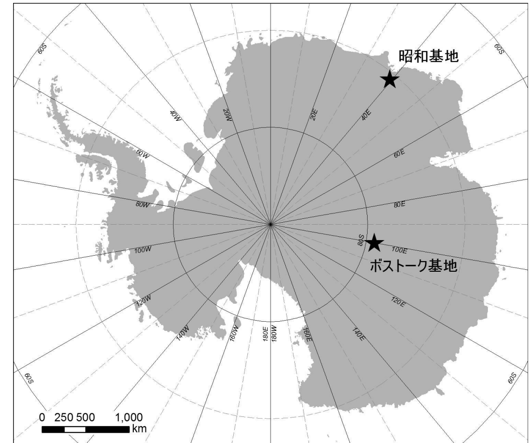
図3 南極大陸
