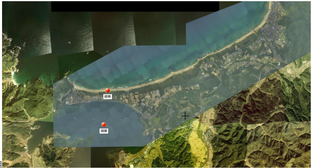
砂州と潟湖
